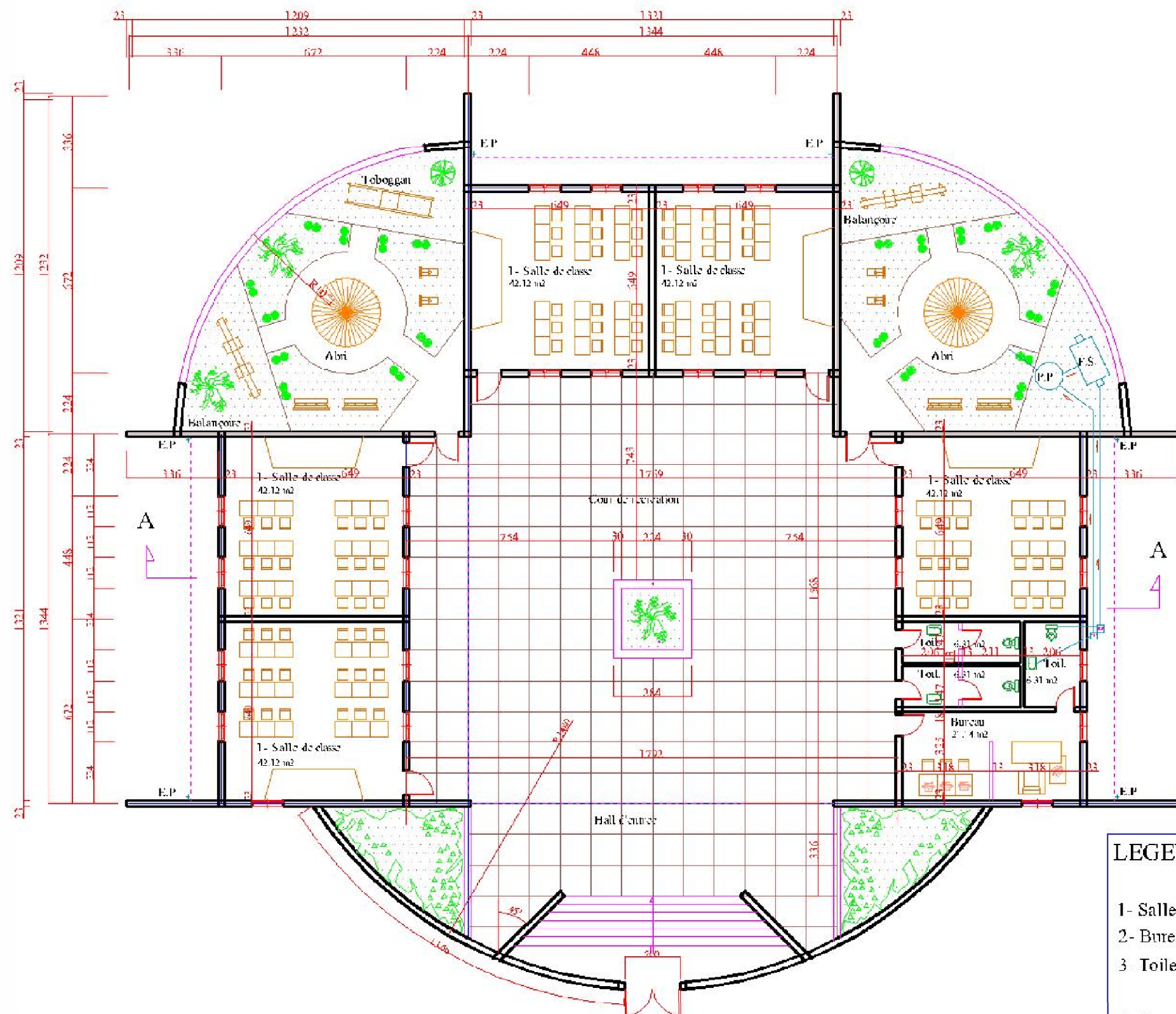
PLAN REZ-DE-CHAUSSEE ECH: 1/200e
