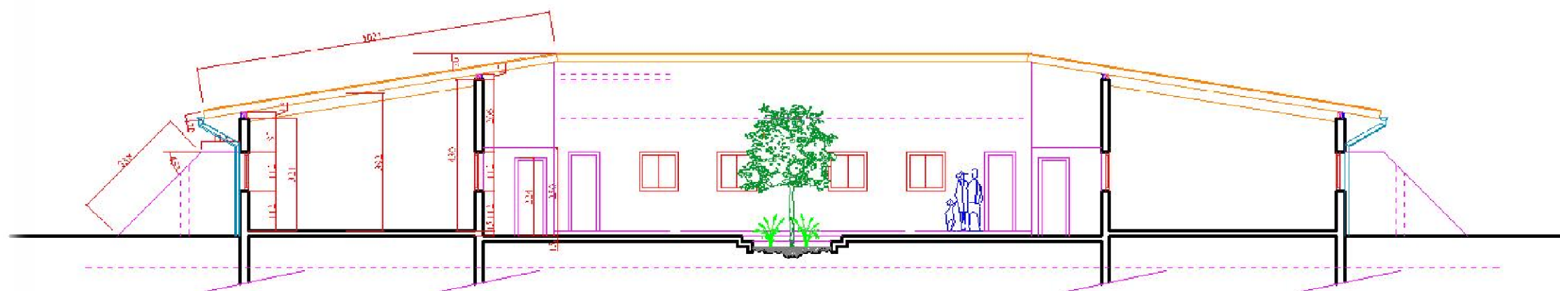
COUPE AA ECH: 1/200e
