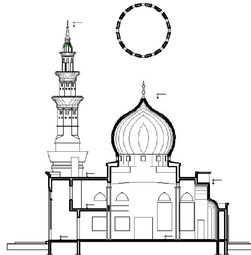
COUPE A.A
