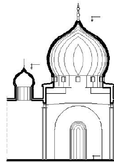
COUPE B.B
